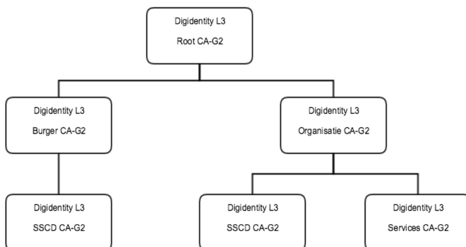
Figuur1.1: Overzicht van de certificaat policies.
